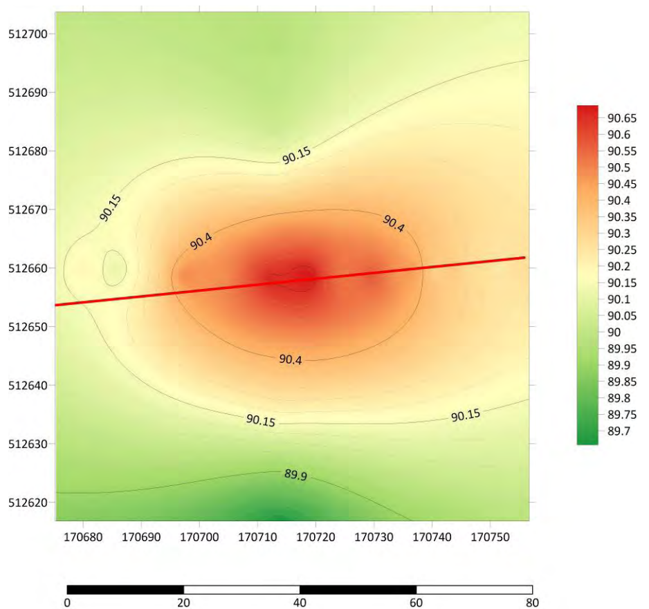
Profilul altimetric
