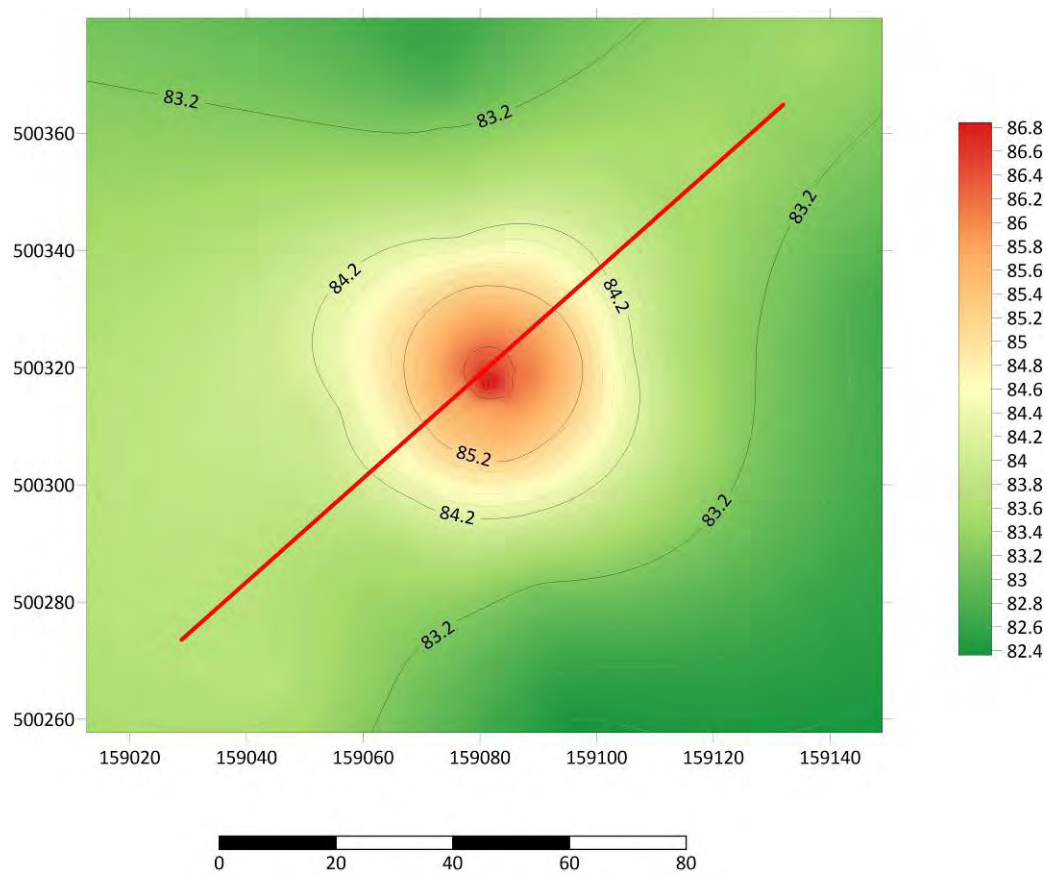
Profilul altimetric
