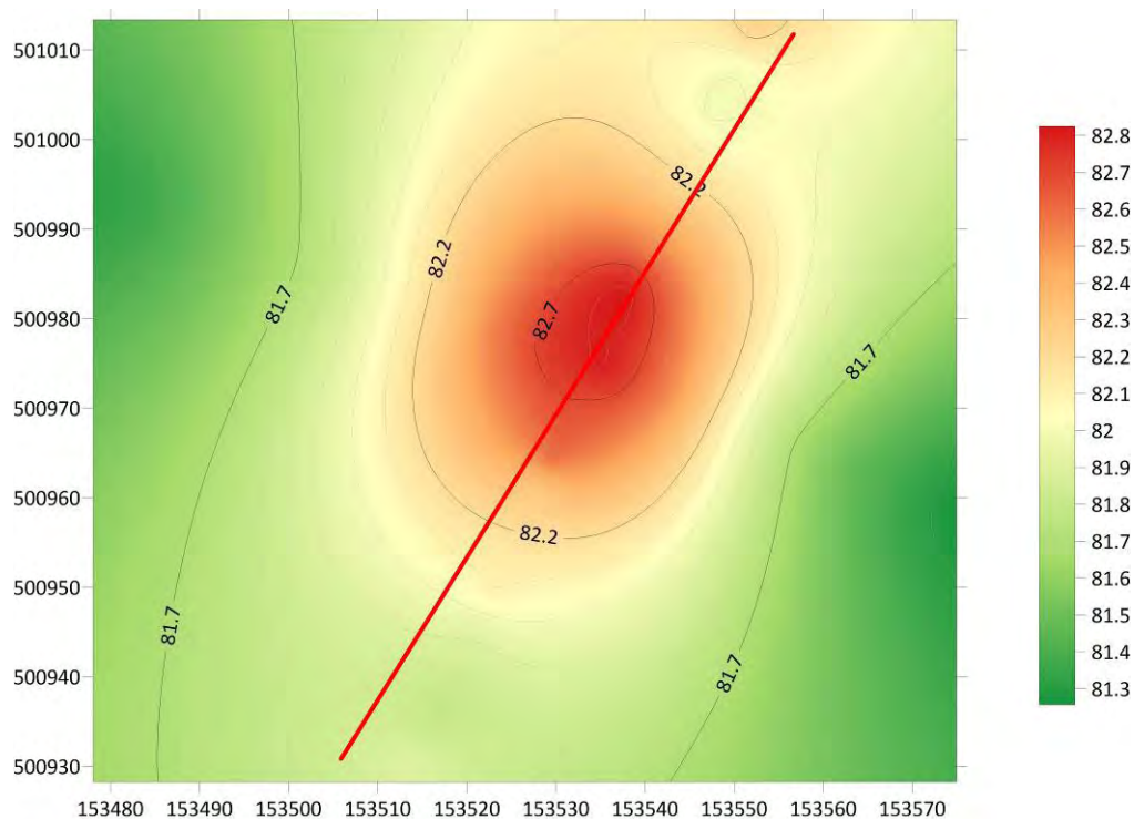
Profilul altimetric
