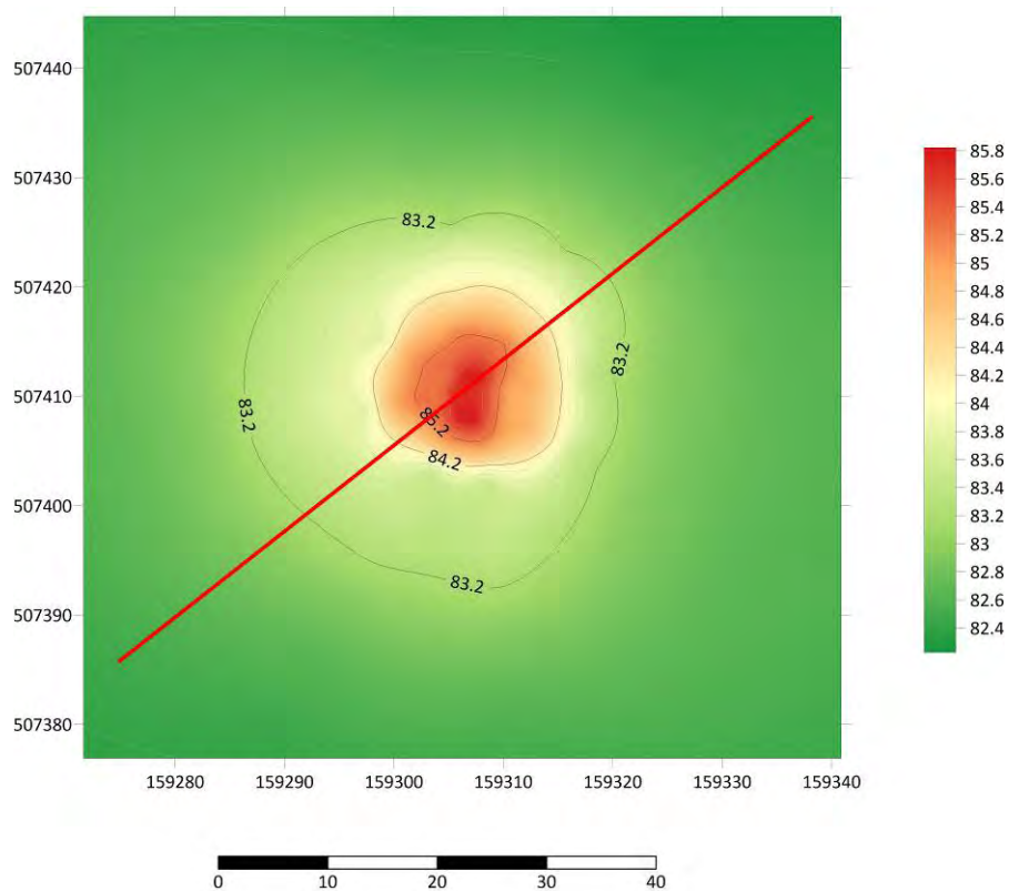
Profilul altimetric
