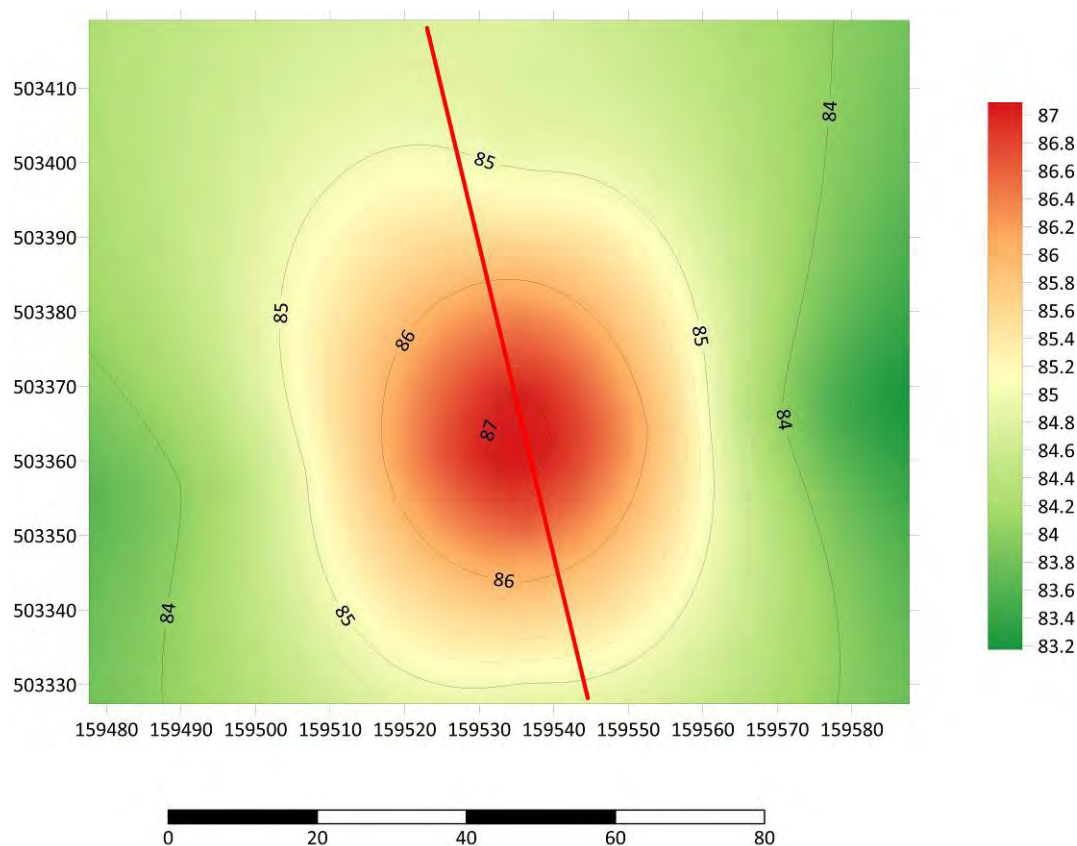
Planul topografic
