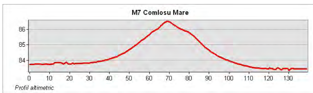
Profilul altimetric
