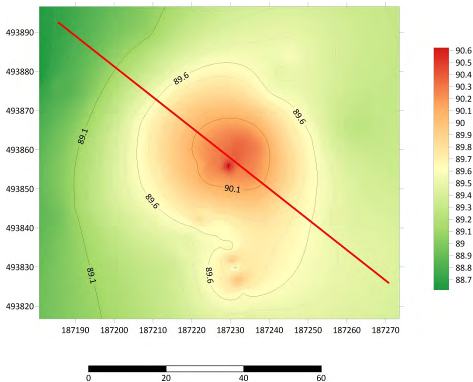
Profilul altimetric
