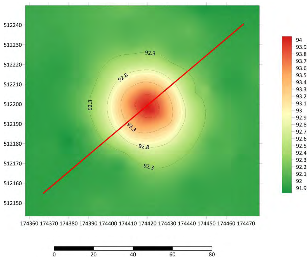
Profilul altimetric
