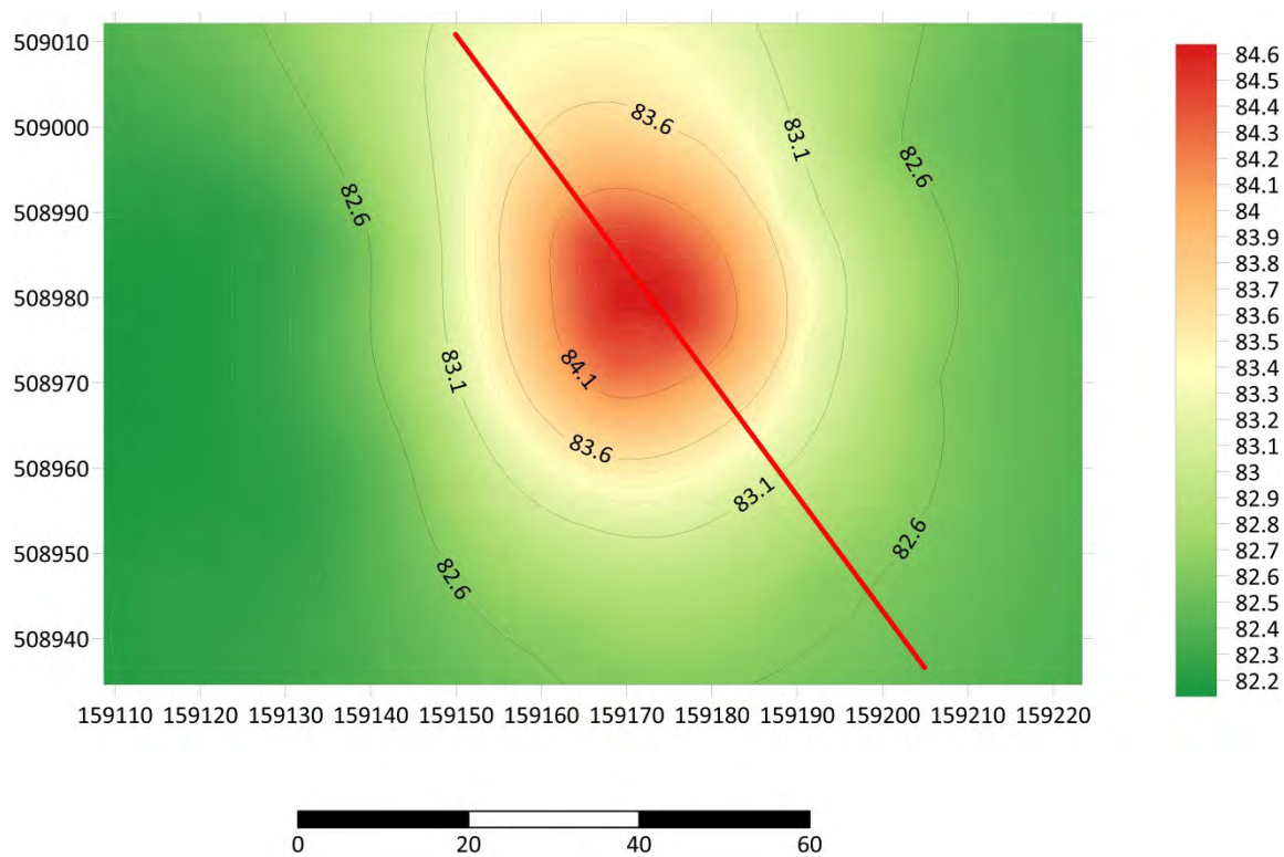
Planul topografic
