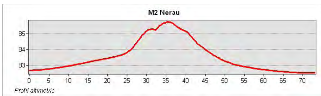
Profilul altimetric
