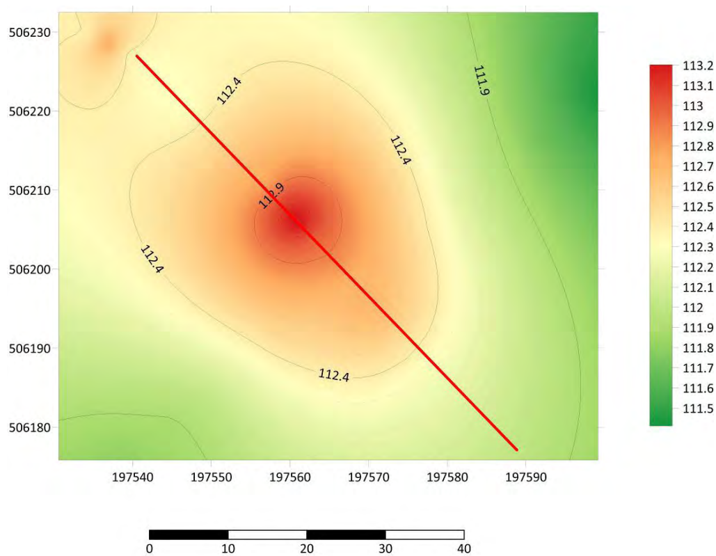
Planul topografic
