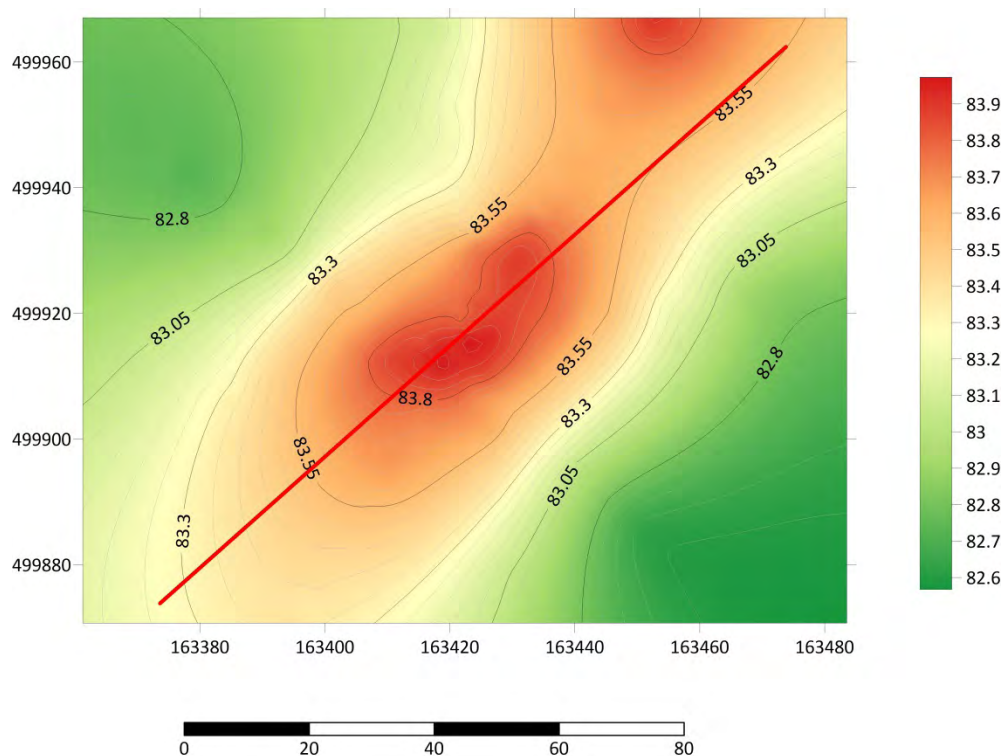
Profilul altimetric
