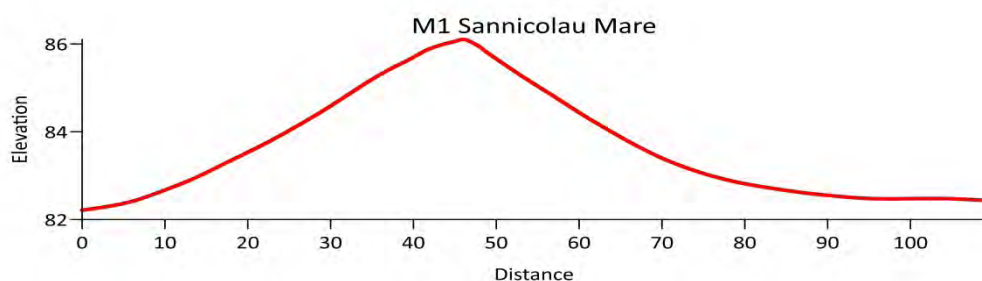
Profilul altimetric
