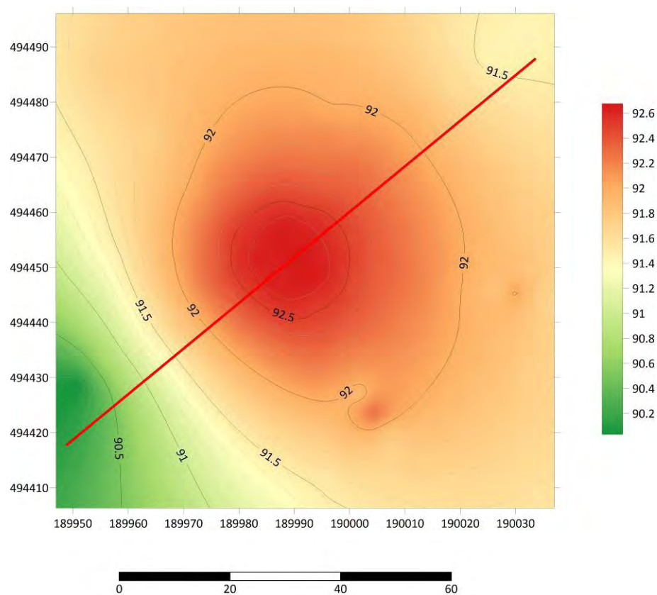
Profilul altimetric
