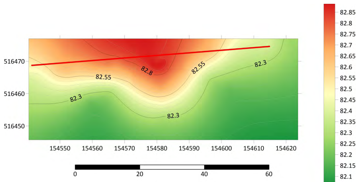
Profilul altimetric
