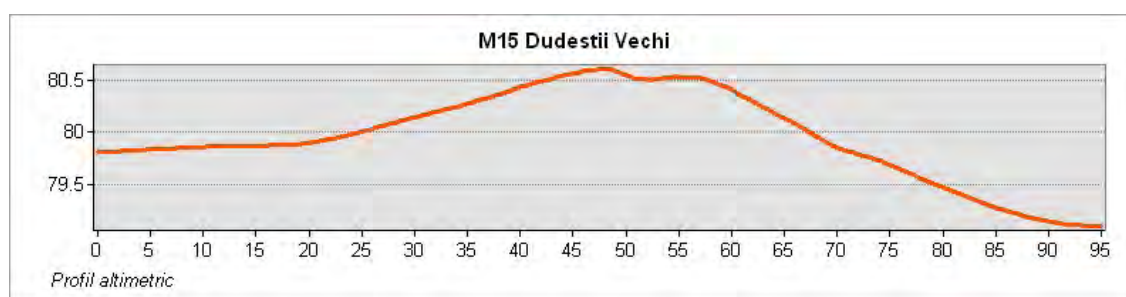
Profilul altimetric
