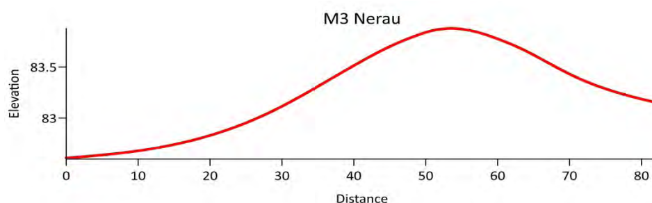
Profilul altimetric
