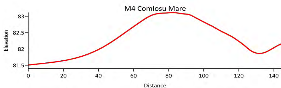
Profilul altimetric
