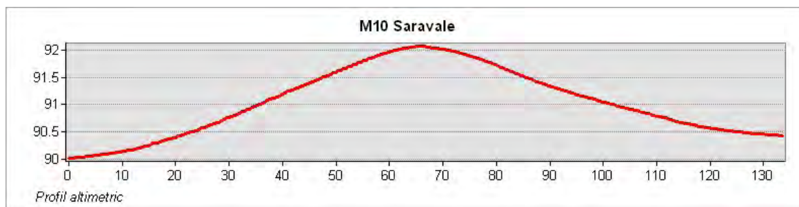
Profilul altimetric
