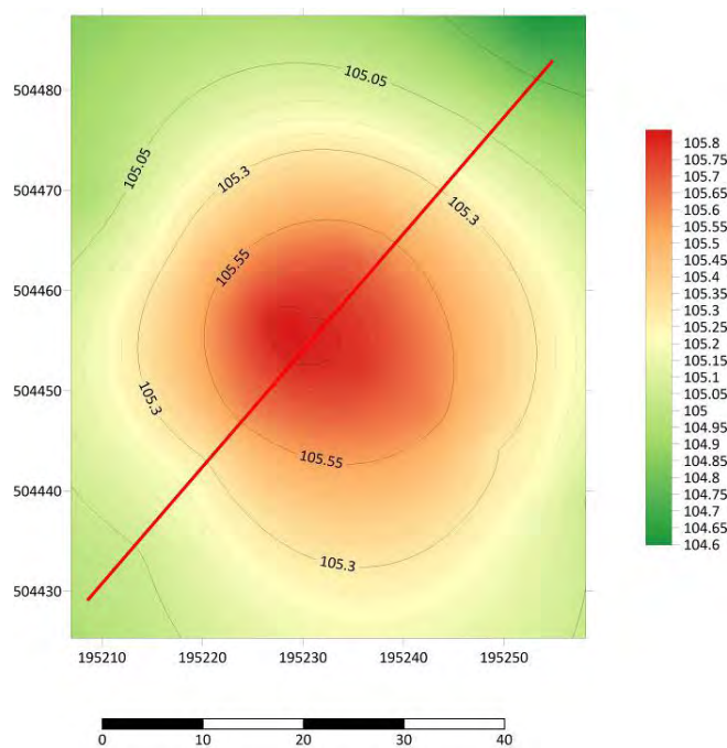
Profilul altimetric
