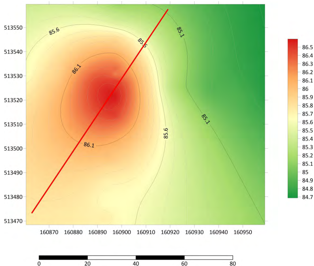
Profilul altimetric
