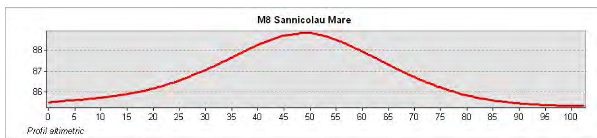
Profilul altimetric
