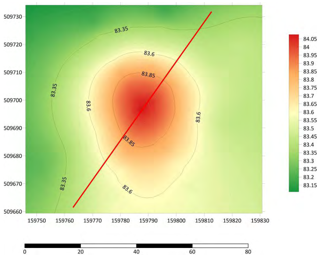
Profilul altimetric
