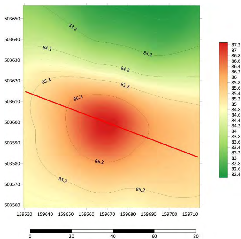
Profilul altimetric
